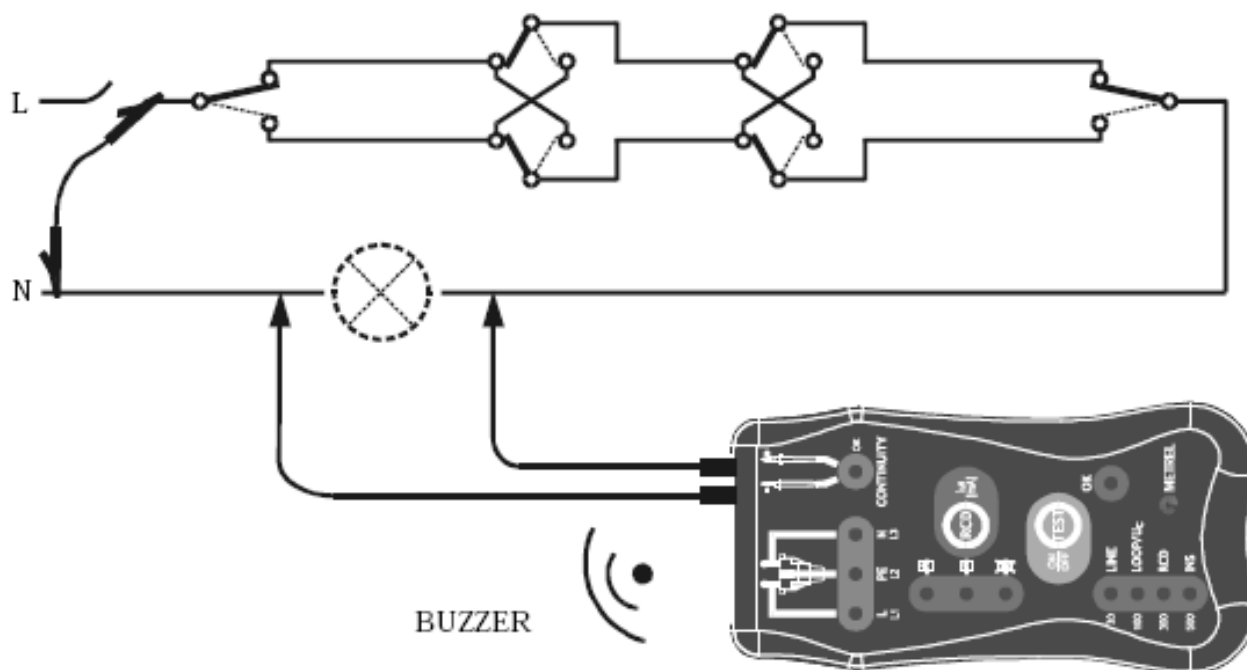
Рисунок. 07 Испытание индикатора цепи электропроводки
