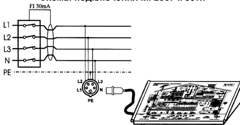
3-х фазная сеть
