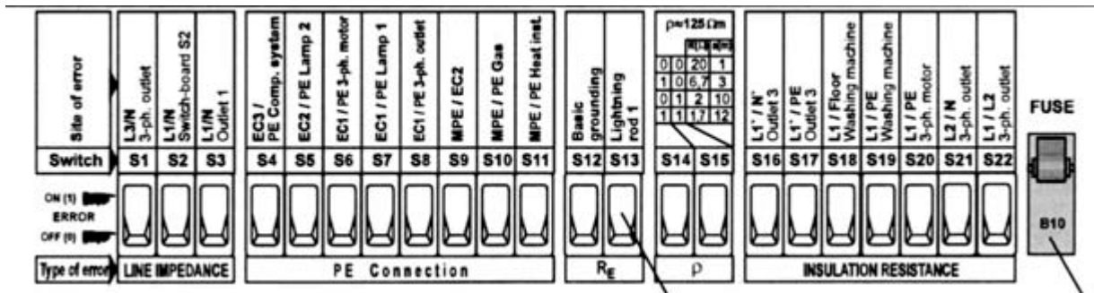
Рис.4. Переключатели (подробнее см. п.8)
