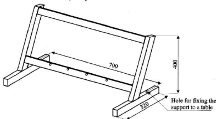
Рис.1. Подставка для стенда
