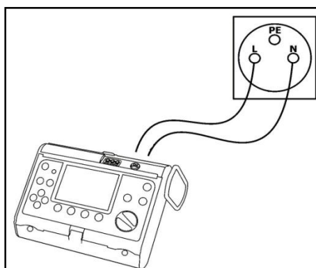
Рис.18. Подключение прибора.
