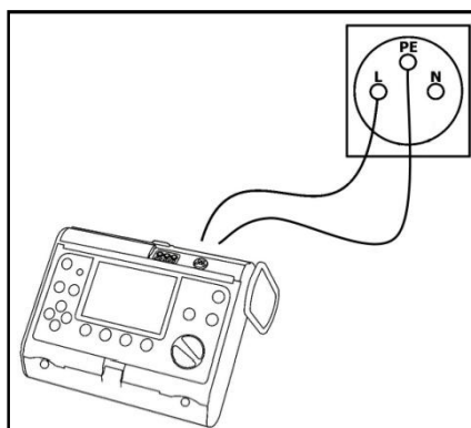
Рис.19. Подключение прибора.
